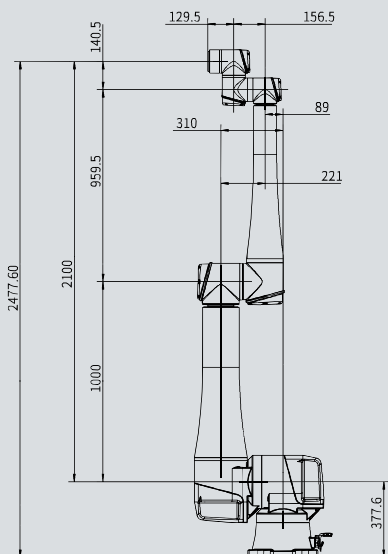
AUBO-iS35 Dimensions
